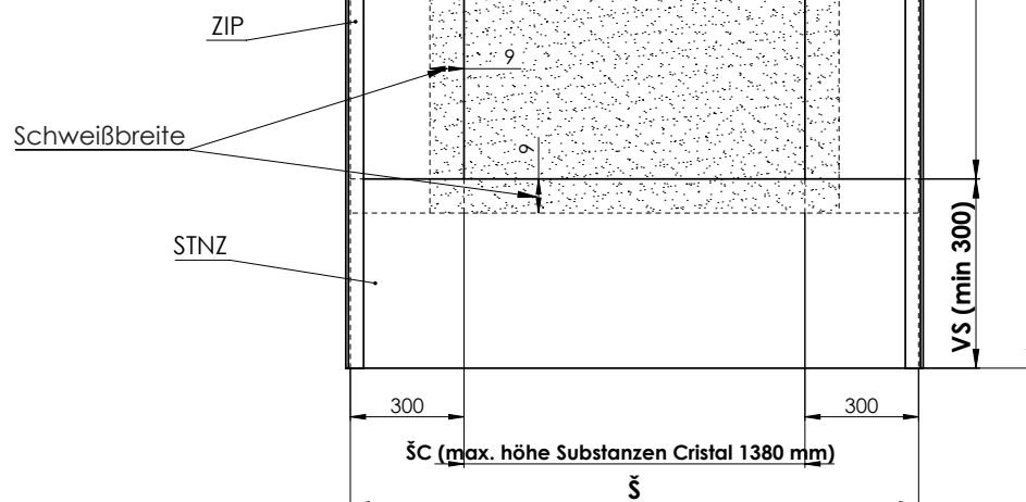
AUSFÜHRUNG DES VERTIKALSTOFFES CRISTAL FÜR PRODUKTE SCREEN ZIP UND SCREEN ZIP ECONOMY
