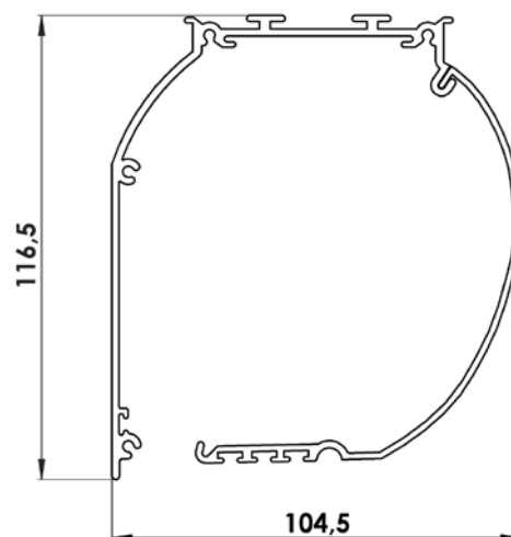
Oberprofil CT 105
