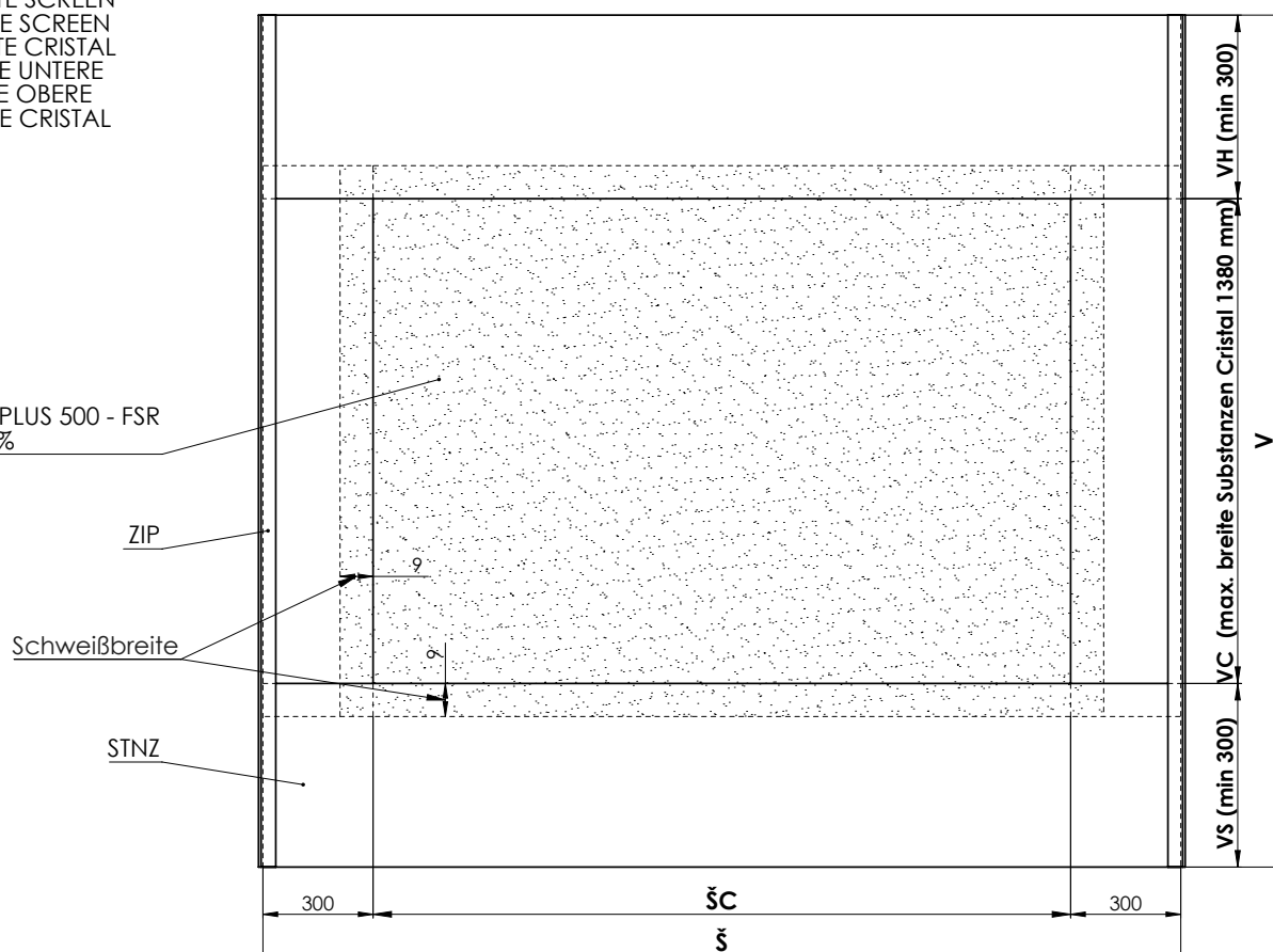
AUSFÜHRUNG DES HORIZONTALSTOFFES CRISTAL FÜR PRODUKTE SCREEN ZIP UND SCREEN ZIP ECONOMY
