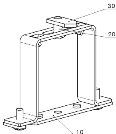
Oberschienenhalter Fe für Heluz P 002/31 (2-01688-0000)
