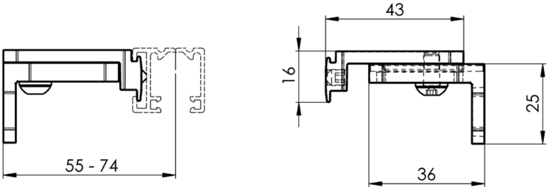
Führungsschienenhalter 055 - 74 mm Zn P021/50 (2-01818-PU11)
