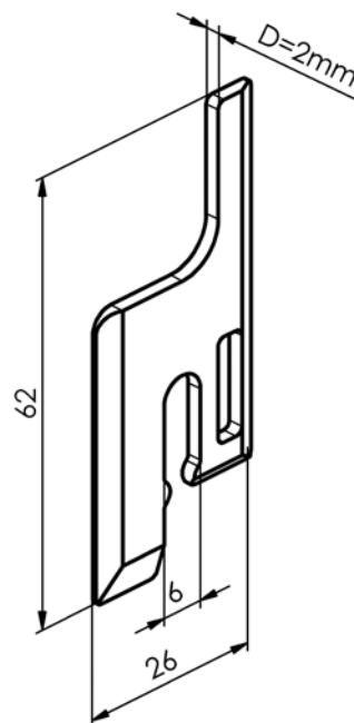
Distanzunterlage P 640 2-02670-XXXX-0
