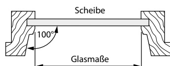
Neue Bauart
