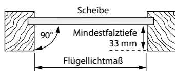
Flügel mit geradem Falz
