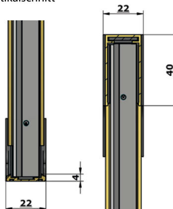
Vertikalschnitt
