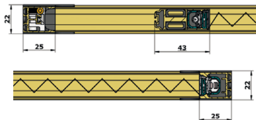
Horizontalschnitt
