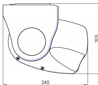
Konsole Decke
