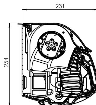
Box mit LED-Beleuchtung
