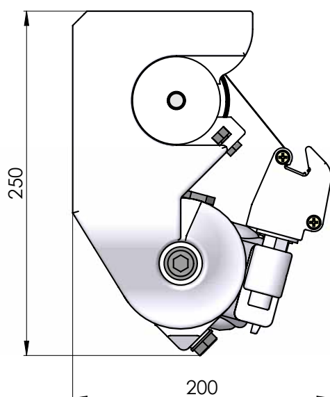
Konsole Wand/Decke
