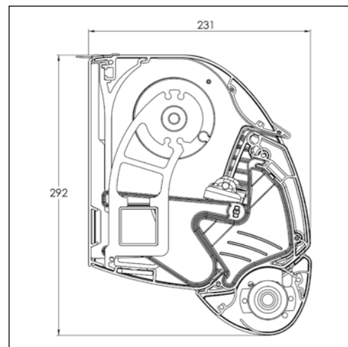
Kastenquerschnitt Olivia mit Variovolant
