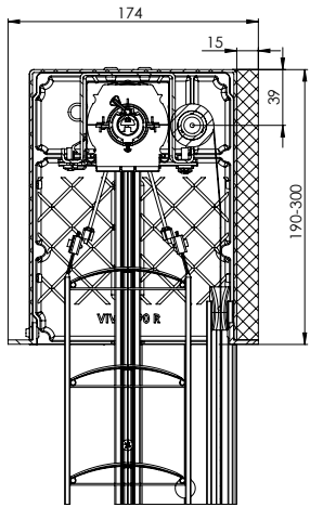
25X15 Extrudiert
